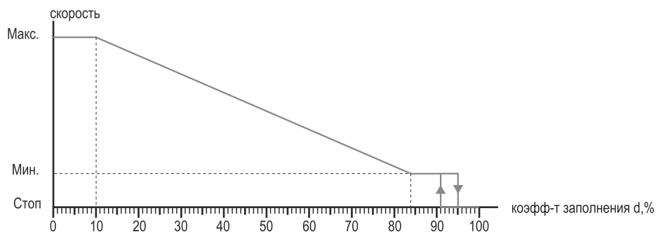
Рис.10 Зависимость скорости от коэффициента заполнения
