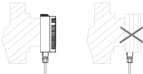
Рис.6 Теплоизоляция насоса
